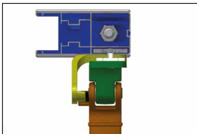
Particolare attacco bracci scorrevoli
