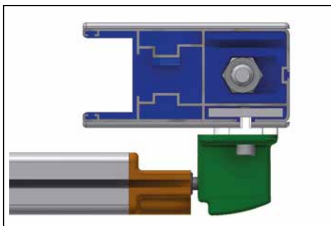
Particolare telo scorrevole
