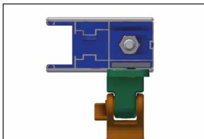
Particolare attacco bracci fissi
