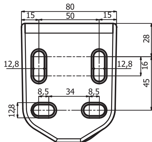
Ingombri e interasse fori installazione a soffitto
