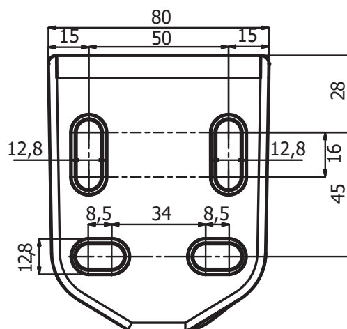
Ingombri e interasse fori installazione a soffitto
