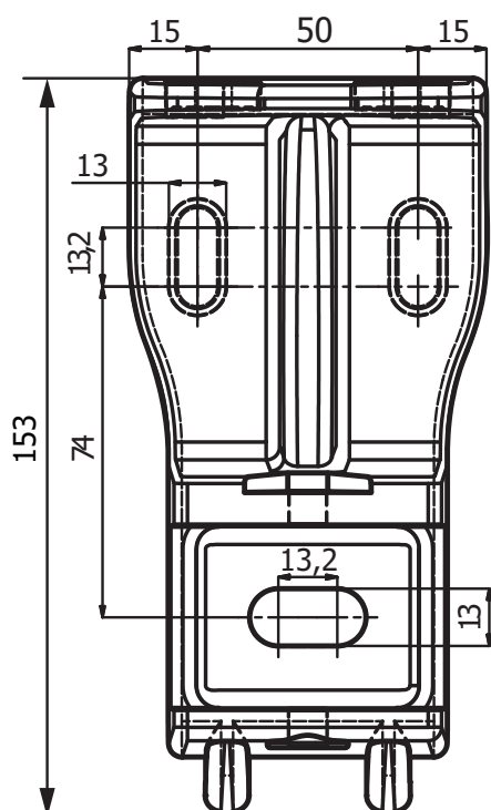
Ingombri e interasse fori installazione a parete
